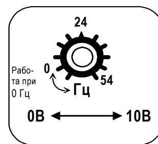
Шкала потенциометра
