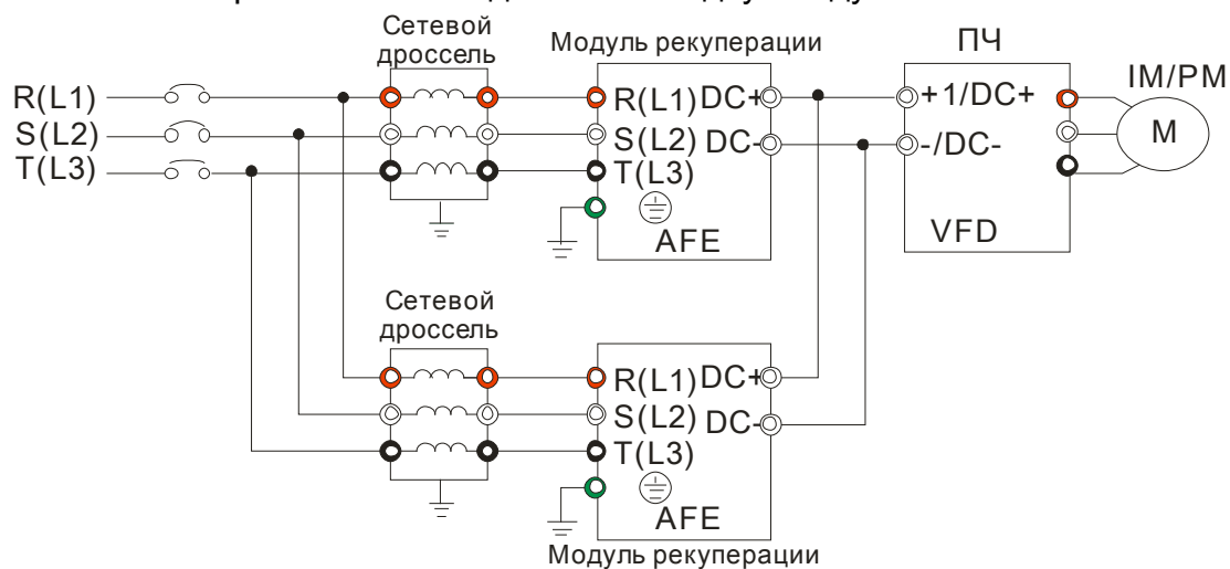
Рисунок 3. Схема подключения при использовании модуля AFE в качестве тормозного модуля
