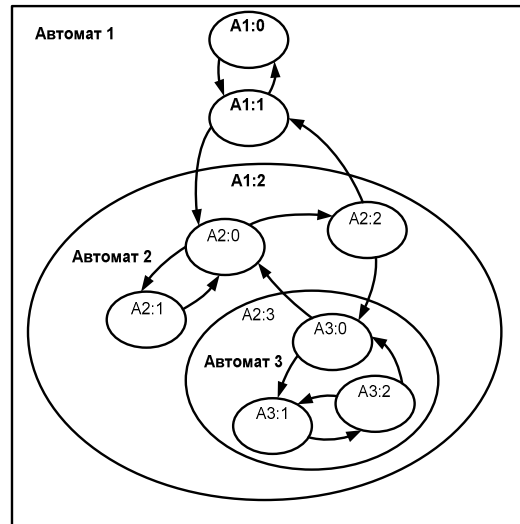
Рис. 3. Вложенные автоматы
