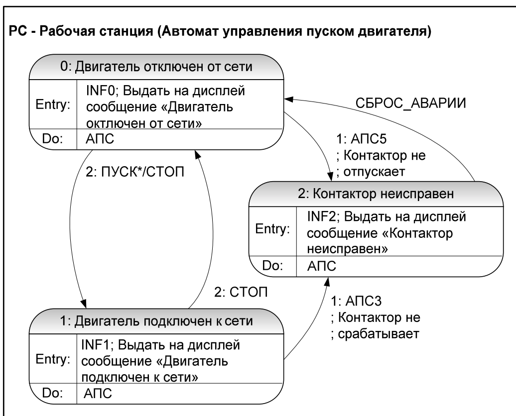
Рис. 6. Граф переходов автомата управления пуском двигателя
